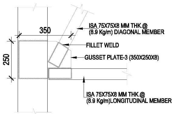
DETAIL - A1
