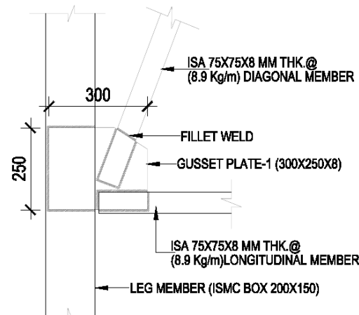
DETAIL - A5
