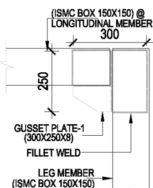
DETAIL - A4
