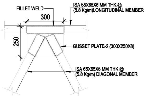
DETAIL - A6
