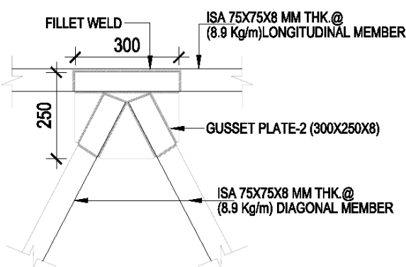
DETAIL - A2
