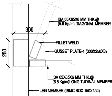
DETAIL - A3
